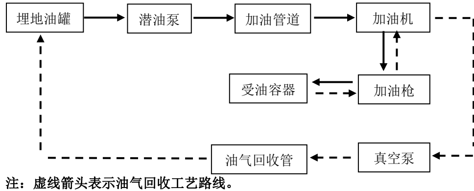
①汽油加油机加油工艺，流程图如下：
