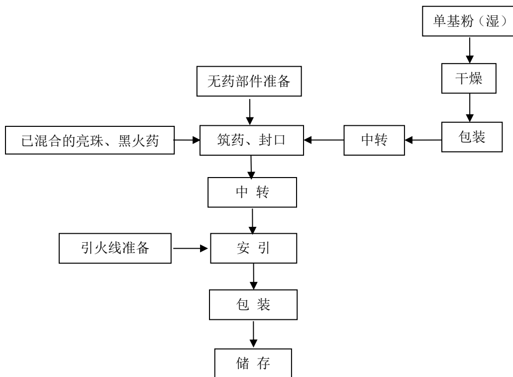
图 2.3-3 吐珠类产品生产工艺流程图
