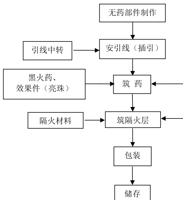
图 2.3-3 吐珠类产品生产工艺流程图
