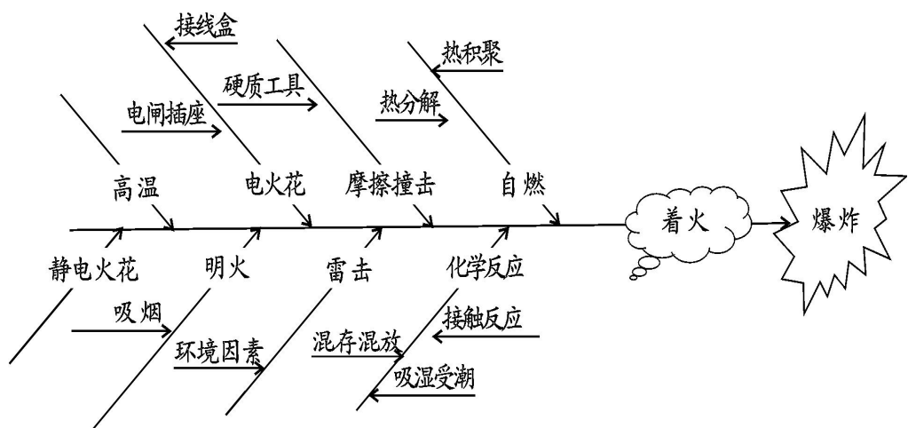
图 3.4-1 烟花爆竹仓库引爆的因果分析图
