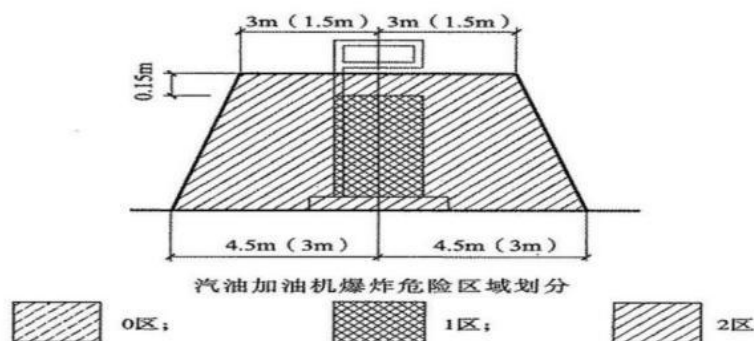
图 3.6-1 汽油加油机爆炸危险区域划分图
