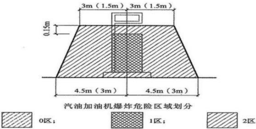
图 3.6-1 汽油加油机爆炸危险区域划分图
