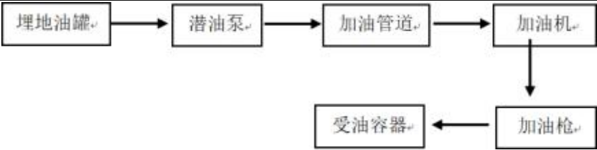
汽油加油机加油工艺框图如下：
