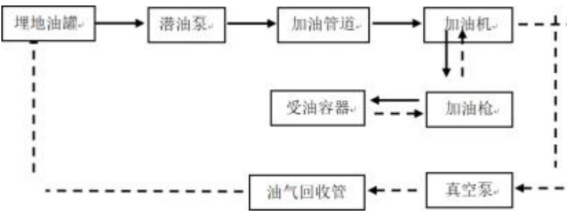
汽油加油机加油工艺框图如下：
