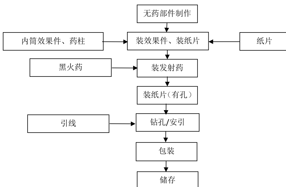
图 2.3-5 小礼花类（圆柱型）产品生产工艺流程图
