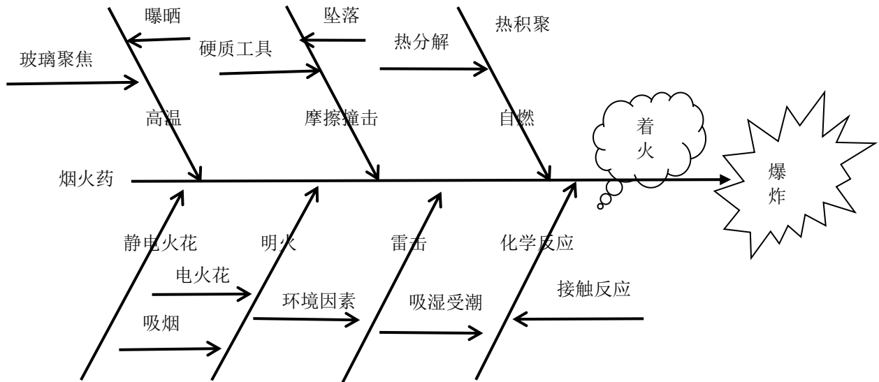
图 3.11-1 燃烧、爆炸触发条件分析图
