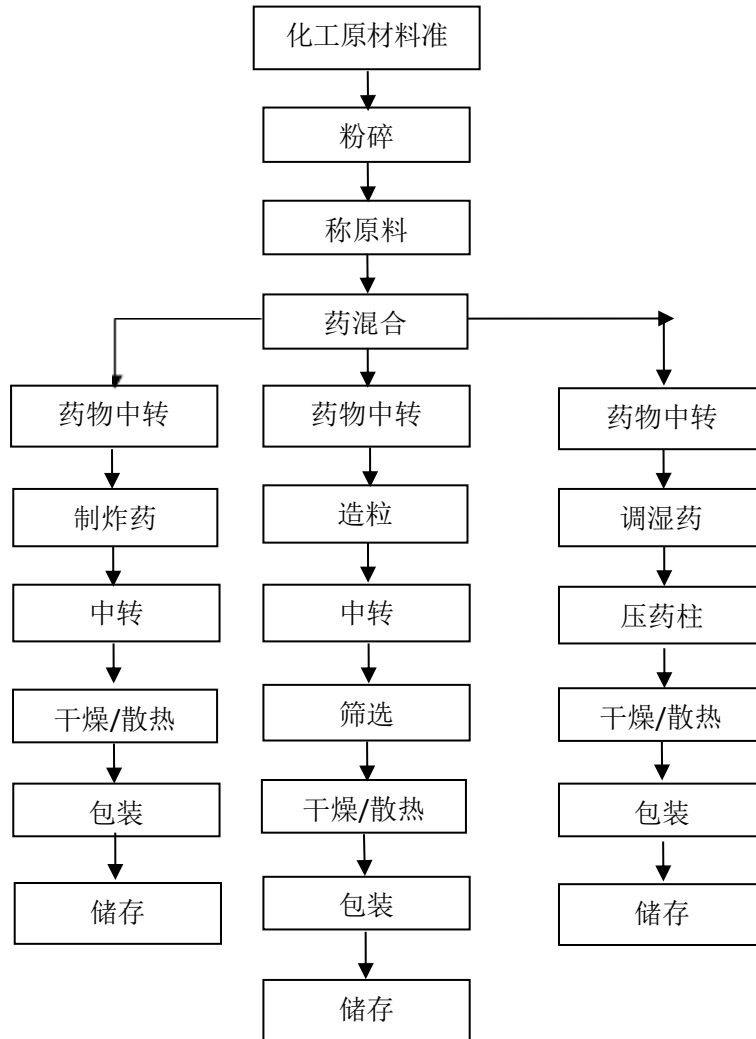
图 2.3-2 药物裸药效果件（炸药、亮珠、药柱）生产工艺流程图
