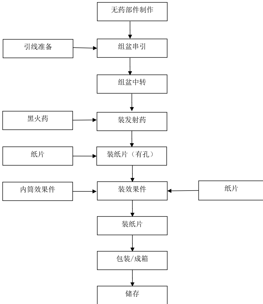
图 2.3-3 组合烟花类产品生产工艺流程图
