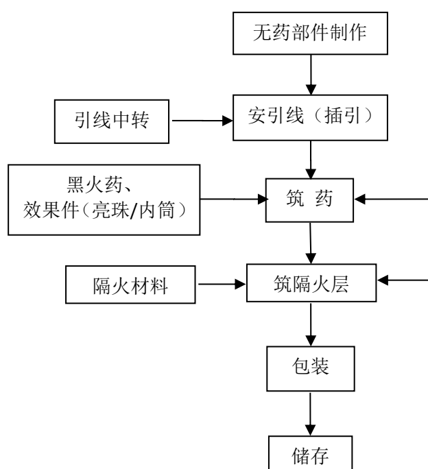
图 2.3-4 吐珠类产品生产工艺流程图
