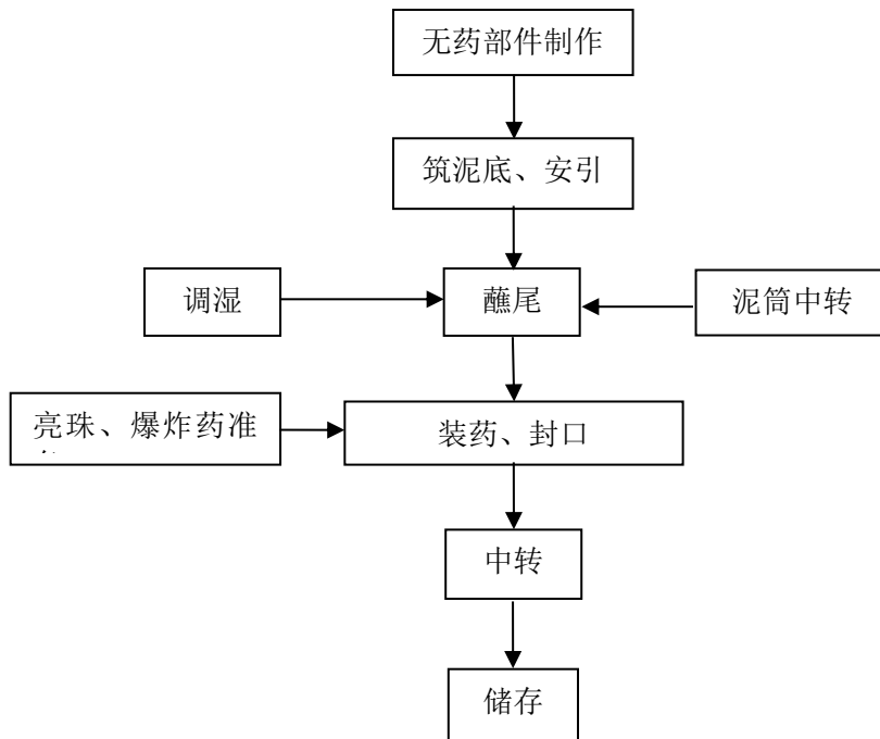
图 2.3-1 效果内筒生产工艺流程图
