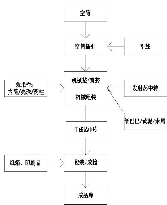
B、C级吐珠类生产工艺流程
