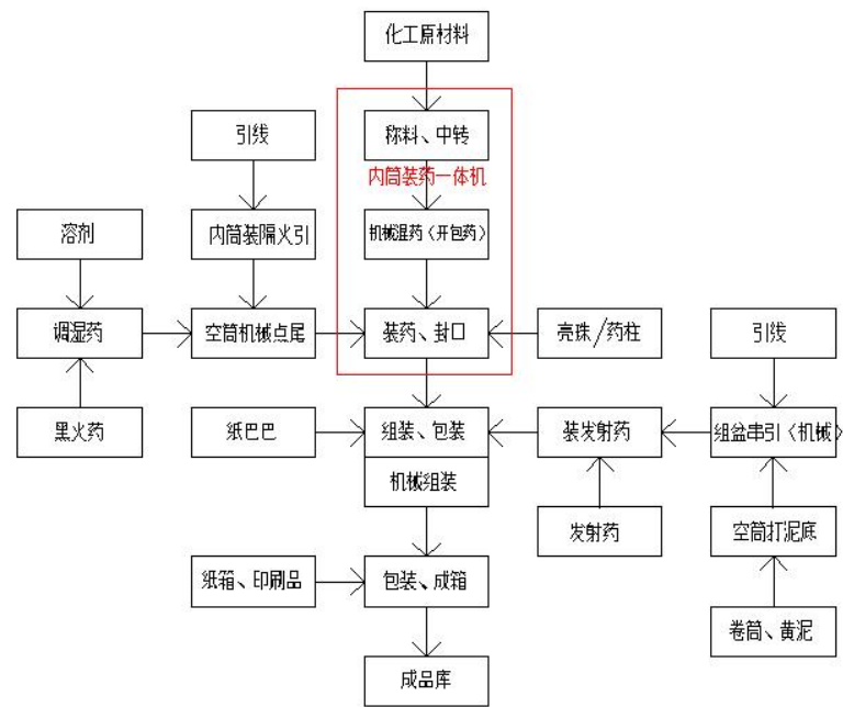
B、C级组合烟花生产工艺流程
