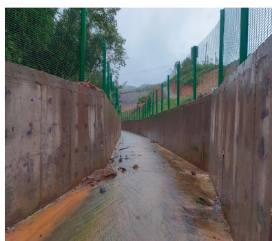
排水明渠
