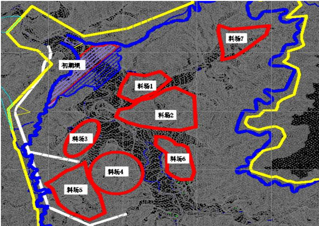
图 2-3 尾矿库料场原拟选位置示意图
