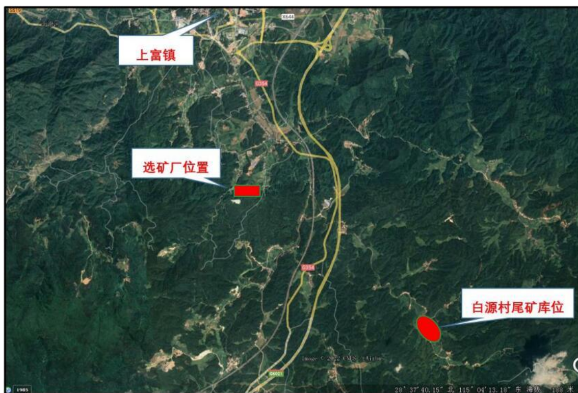
图 2-2 尾矿库、选矿厂相对位置示意图
